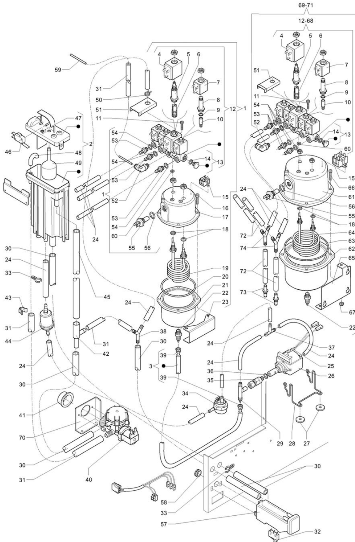
Tavola :05 - Circuito idraulico
