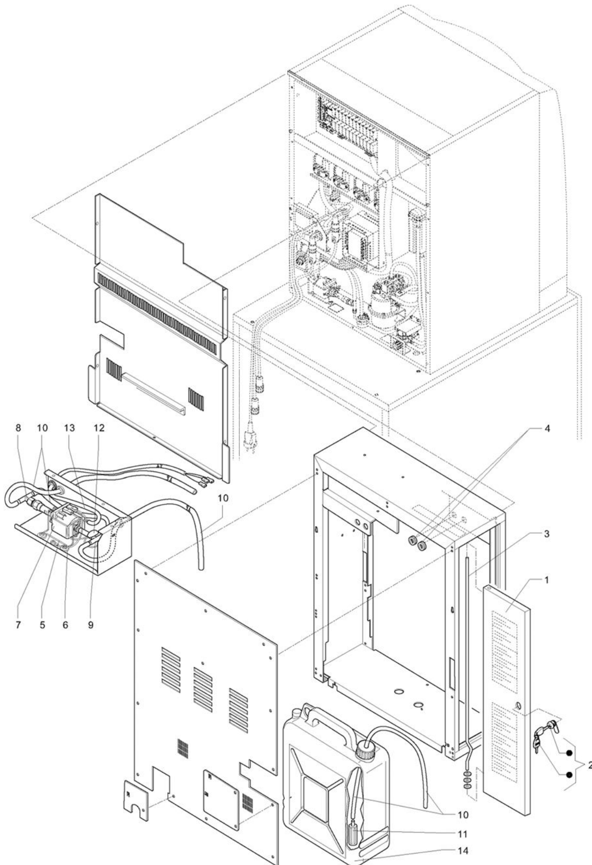
Tavola :15 - Modulo posteriore
