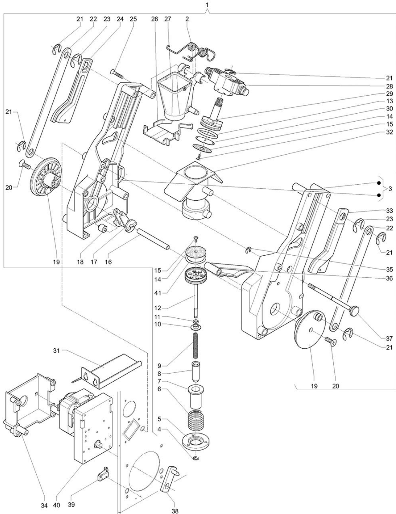
Tavola :10 - Gruppo caffè
