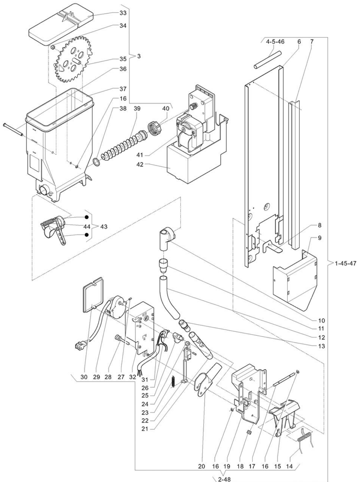
Tavola :07 - Distributore zucchero/nalette
