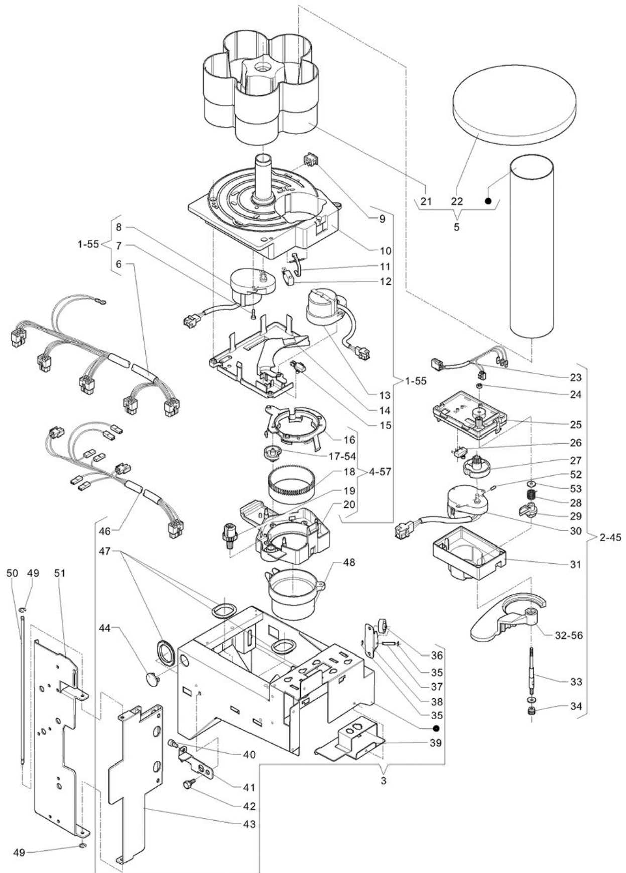
Tavola :06 - Distributore bicchieri
