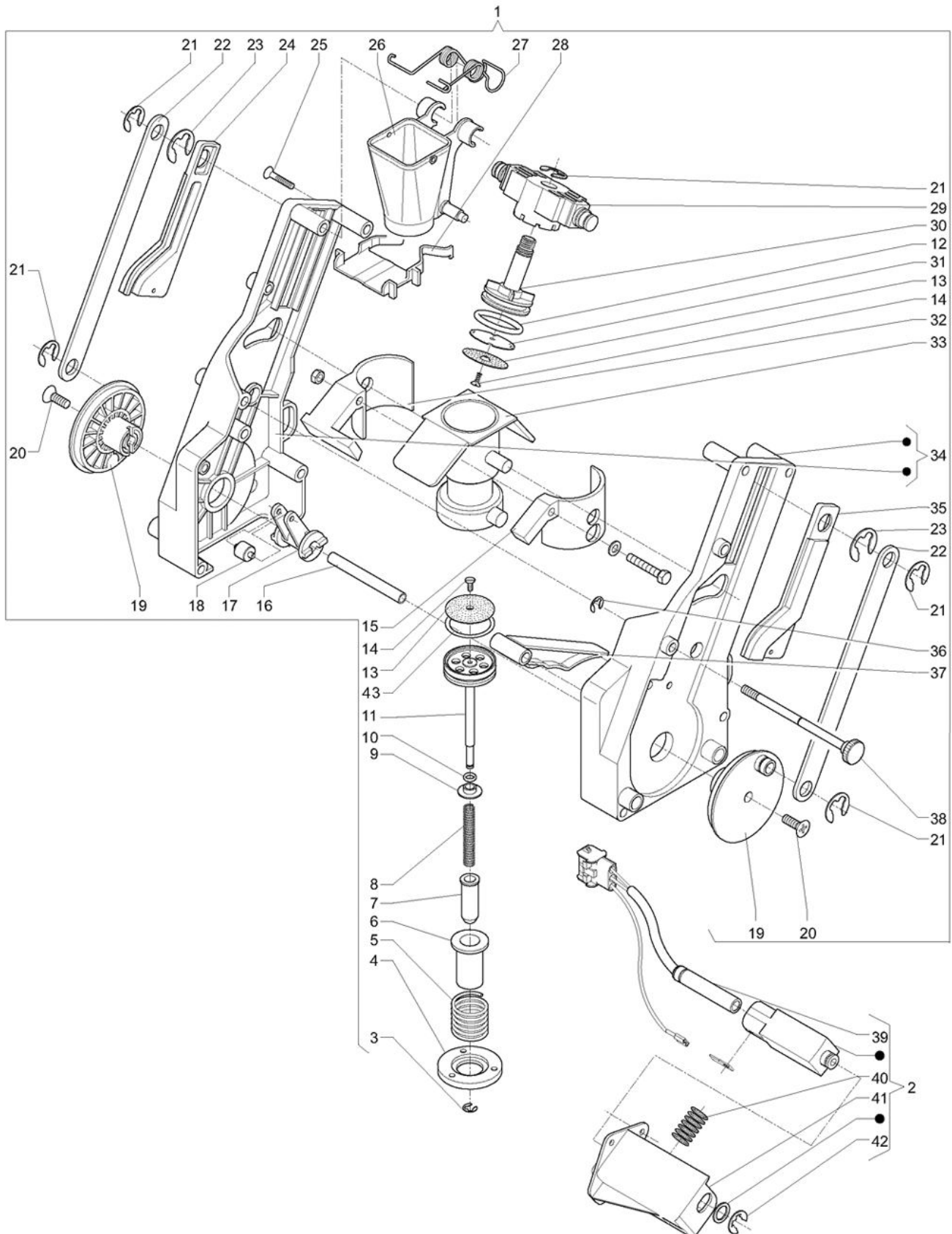
Tavola :11 - Gruppo caffè (in apertura)
