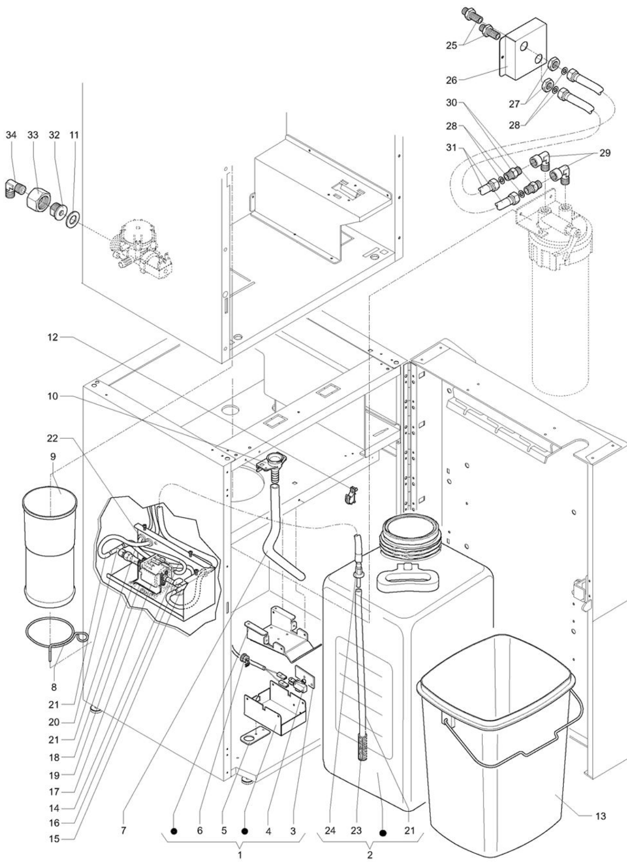
Tavola :14 - Mobilietto e kits
