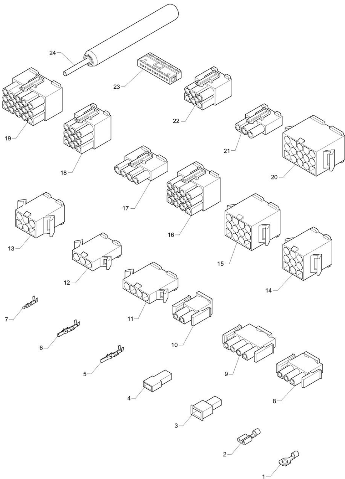
Tavola :16 - Connettori e terminali
